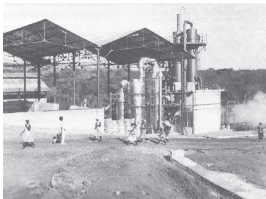
Photo 2: Premier atelier de fabrication d'acide sulfurique
